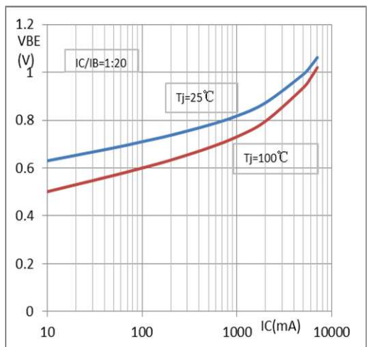
V_{BE(sat)} - I_C
