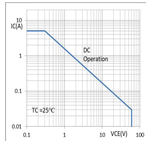
SOA
